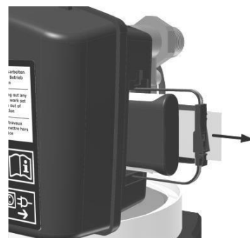
2. Akku mit Lasche herausziehen
