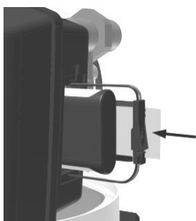
5. Neuen Akku vorsichtig in das Steuerungsgehäuse einführen
